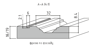
Возможный вариант профиля «по фасаду»
