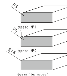
Возможный вариант профиля «по торцу»
