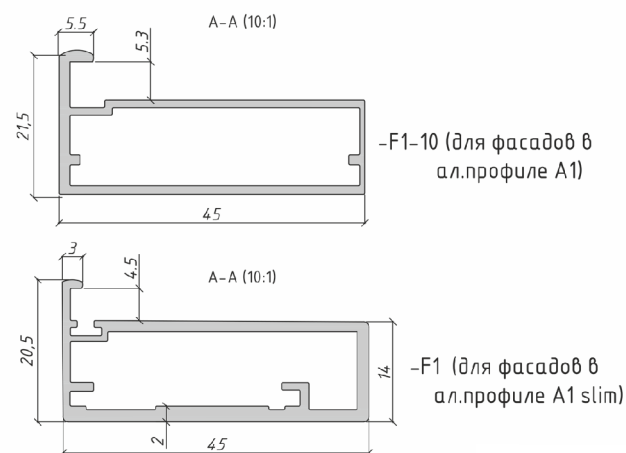
Виды алюминиевых профилей для изготовления рамок с основными техническими параметрами
