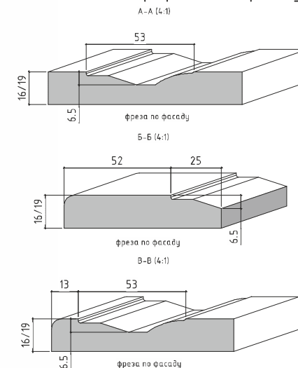
Возможный вариант профиля «по фасаду»
