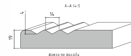
Возможный вариант профиля «по фасаду»
