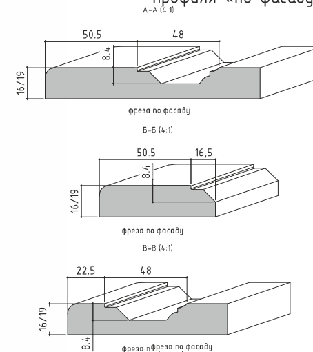
Возможный вариант профиля «по фасаду»
