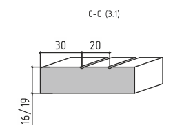
Возможный вариант профиля по торцу
