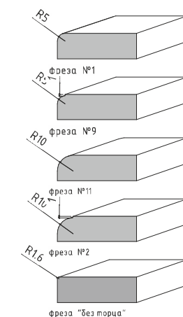
Возможный вариант профиля «по торцу»
