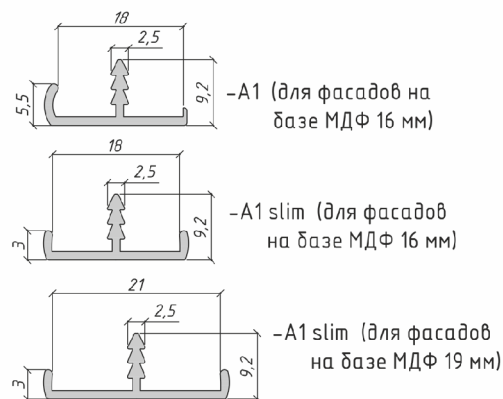
Виды алюминиевого профиля с основными техническими параметрами
