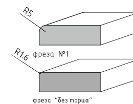
Возможный вариант профиля «по торцу»
