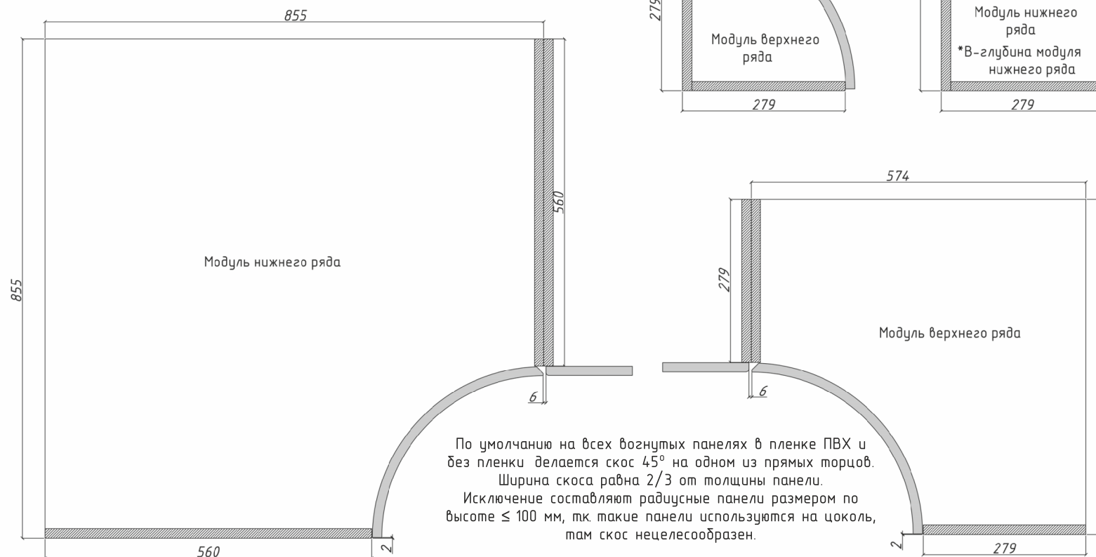
Выгнутый глухой Выгнутый витрина Вогнутый глухой ВНИМАНИЕ! Фрезеровка наносится на выгнутые и вогнутые фасады высотой >250 мм
